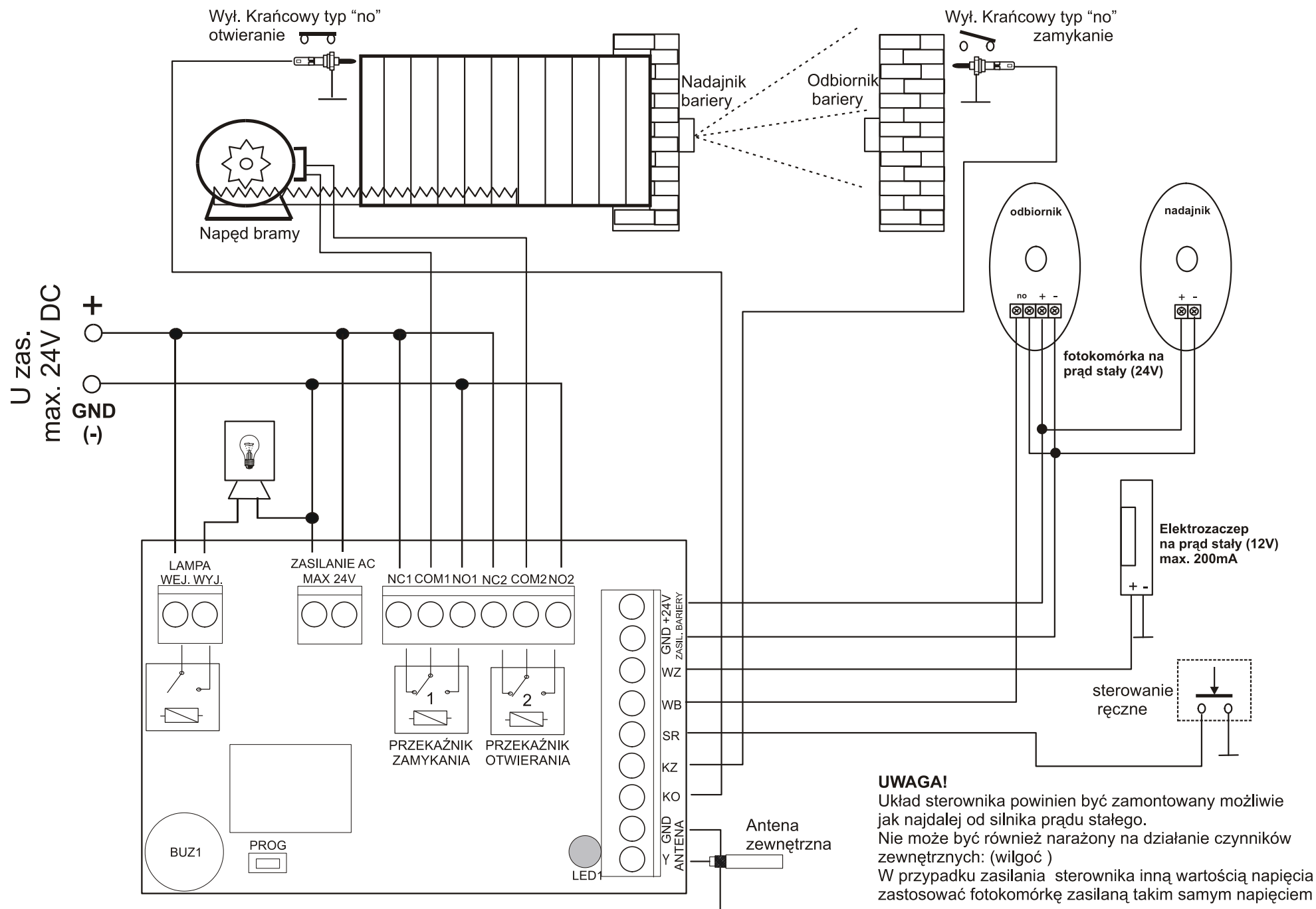
Rys.2 Przykład połączenia sterownika do napędu zasilanego prądem stałym max. 24V
