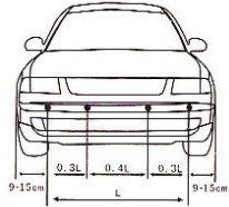
Punkty wiercenia dla czujników.
