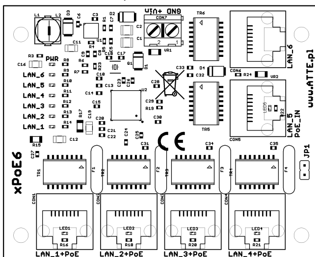
Rys. 1. BCS-xPoE6 - widok zewnętrzny
