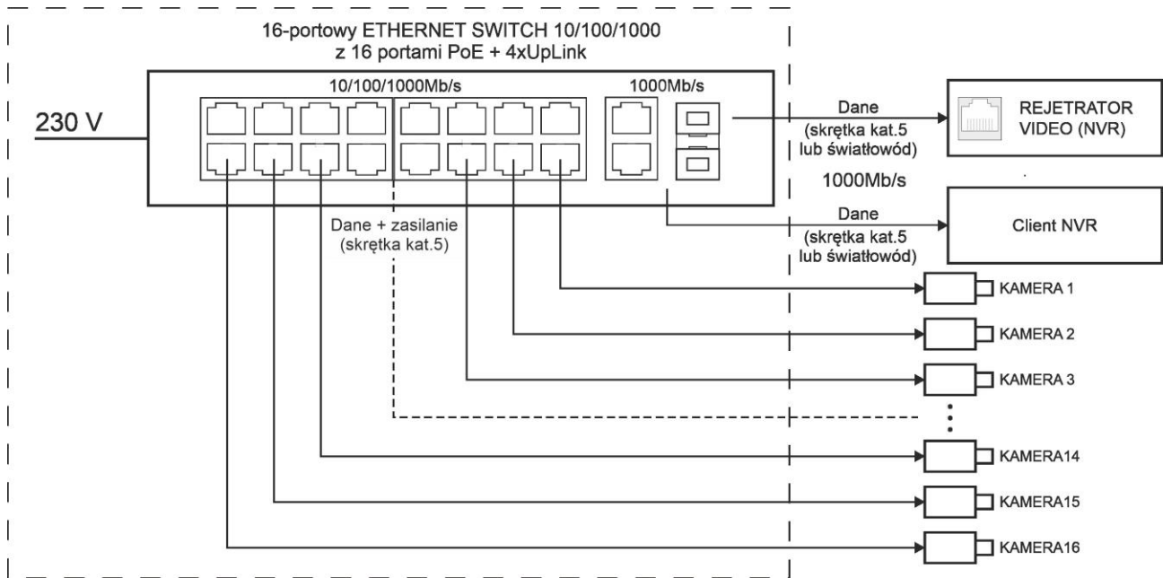
Rys. 1. Schemat blokowy.
