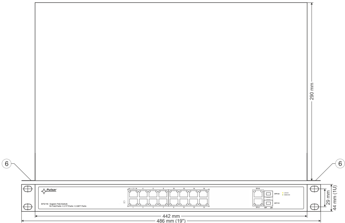
Rys. 4. Widok switch'a.
