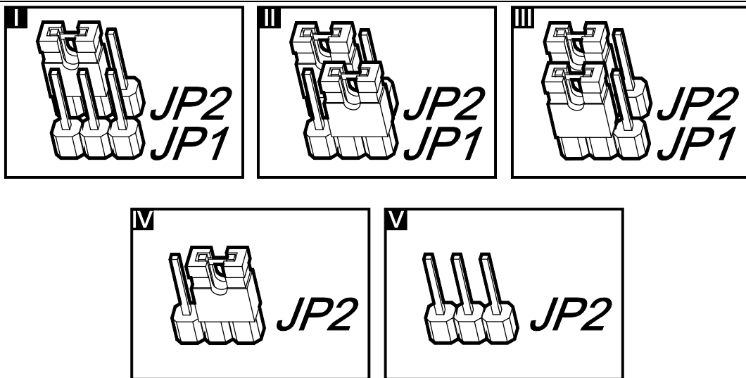
Rys. 3. Sposób zakładania zworek dla uzyskania określonego typu sygnalizacji optycznej.
